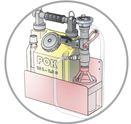
"Handy-foam" avec support en alliage d'aluminium, équipé d'une lance bas foisonnement et d'une lance moyen foisonnement
